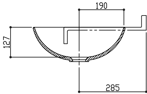
A-A 断面
