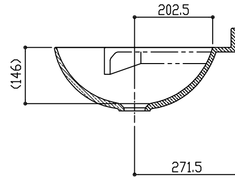
A-A 断面
