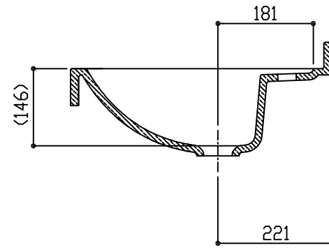
A-A 断面
